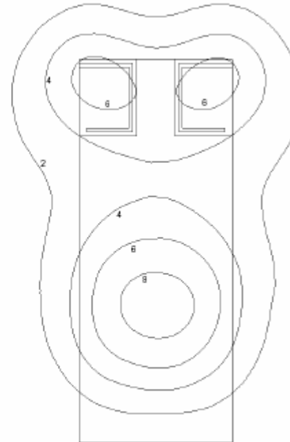
b) DCS 1800
