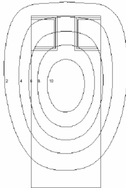
a) GSM 900
