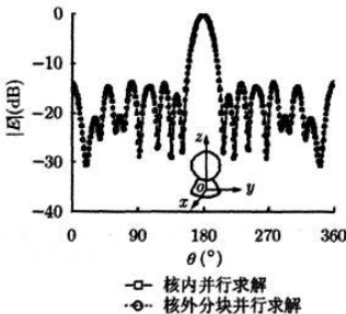
图 8 金属组合体归一化散射方向图
