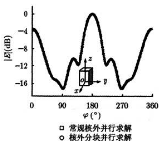
图 7 金属立方体归一化散射方向图
