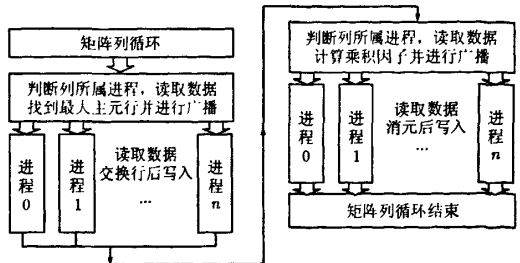
图 4 核外并行消元过程
