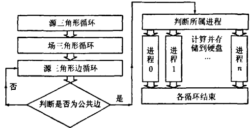
图 3 核外并行矩阵填充
