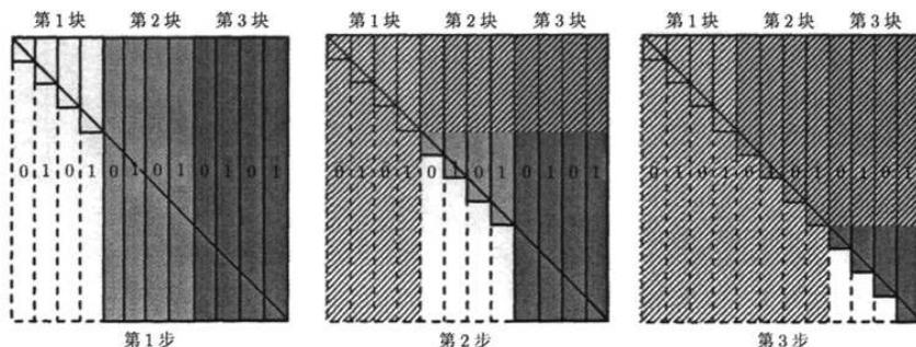
图6 核外分块并行高斯消元示意图
