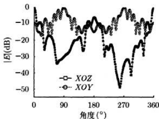
图10 飞机模型归一化散射方向图
