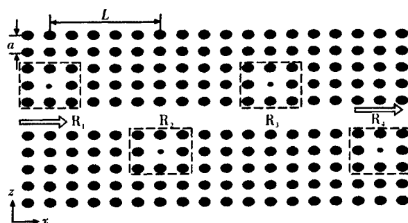
图1 由光子晶体波导和 N 个周期排列的谐振腔组成的滤波器示意图
