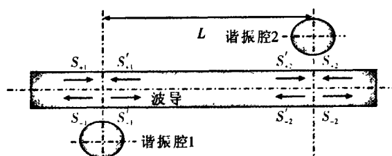
图2 波导和两个谐振腔耦合的基本结构
