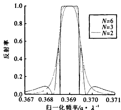
(c) N 不同 ( \Phi = \pi/2, Q=1000 )
