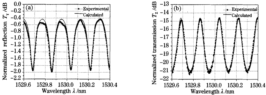
图 2 跑道形谐振腔的输出谱形。(a)Y 端口的输出谱,(b)Z 端口的输出谱
