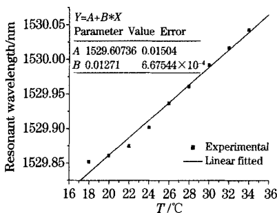
图 3 谐振波长的漂移随温度变化的关系
