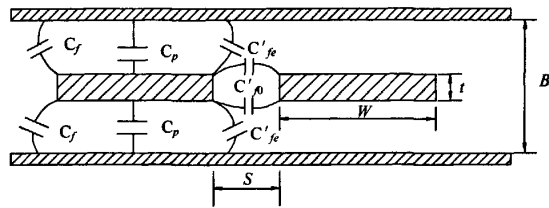
图2 平行耦合矩形杆的各边缘电容和平板电容
