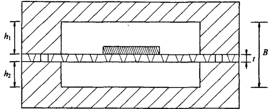
图 3 悬置线内部尺寸
