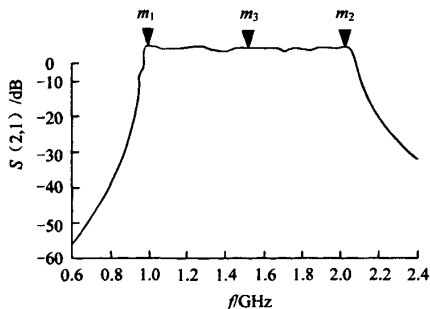
(a) ADS 仿真的频带响应
