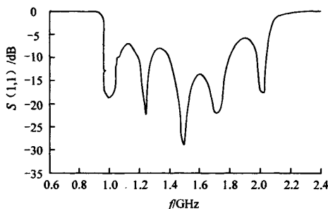
(b) ADS 仿真反射系数响应
