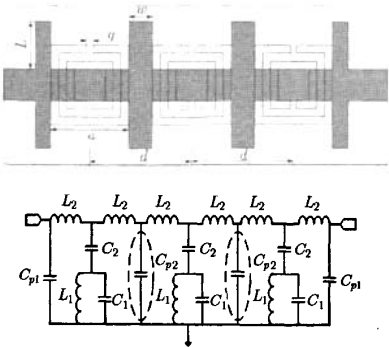
图 6 三单元级联SRR DGS 及其等效电路 ( w=4\text{ mm} , L=9\text{ mm} , d=14\text{ mm} , C_{p1}=1.475\text{ pF} , C_{p2}=2.509\text{ pF} )
