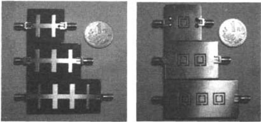
图 8 不同单元数 SRR DGS 实物图
