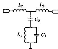
(b) SRR DGS 单元等效电路
