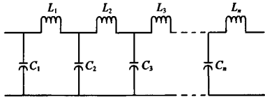
图 1 低通滤波器等效电路
