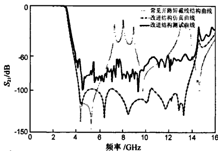
图 6 结果曲线对比图
