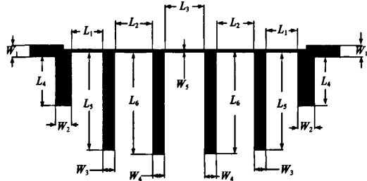
图 2 常见开路短截线结构
