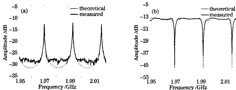
图 6 可调的光学延时器增大 250 ps 时,理论计算和实验测量滤波器频率响应曲线图(a)可调谐滤波器 T_2 的中心波长对准抽运光波长(b)可调谐滤波器 T_2 的中心波长偏离抽运光波长 0.24 nm
