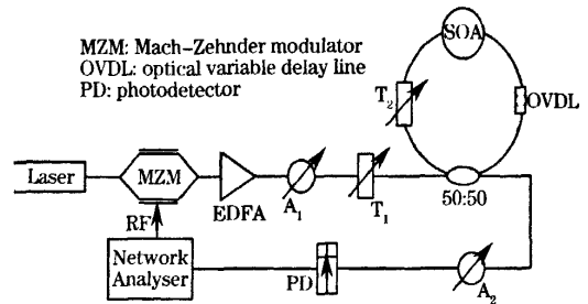
图 1 全光微波滤波器的结构示意图
