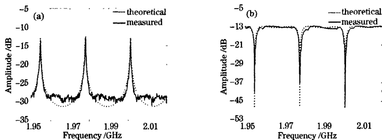
图5 可调的光学延时器置为零时,理论计算和实验测量滤波器频率响应曲线图(a)可调谐滤波器 T_2 的中心波长
