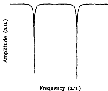
图3 平通带陷波滤波器
