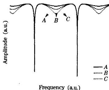
图4 通带平坦度随着 R_1 的变大而变差
