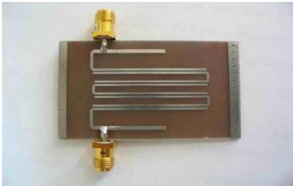
图 3 滤波器实物照像
