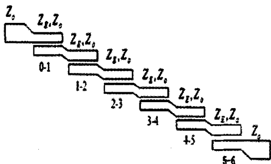
图 1 5 阶带通滤波电路
