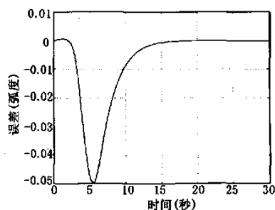
图6 台体机动时天线的跟踪误差曲线图
