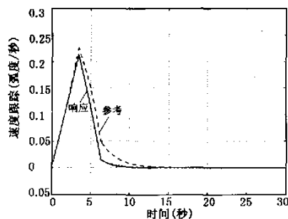
图5 台体机动时天线的速度跟踪曲线图
