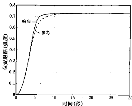
图 4 台体机动时天线的位置跟踪曲线图
