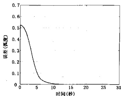
图 3 天线指令跟踪时台体的误差曲线图
