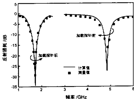
图 3 微带天线输入端反射损耗
