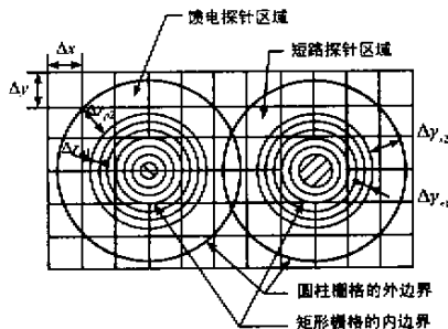
图 2 局部内共形 FDTD 栅格示意图
