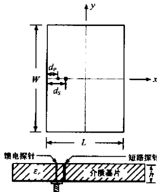
图1 短路探针加载微带贴片天线
