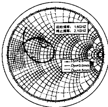
图 4 输入阻抗随 D_p 的变化
