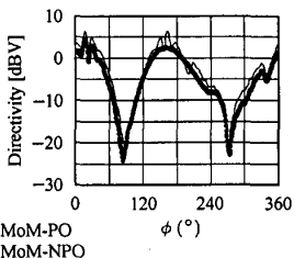
图6 x - y 面的方向性比较 Fig.6 Directivity on x - y plane
