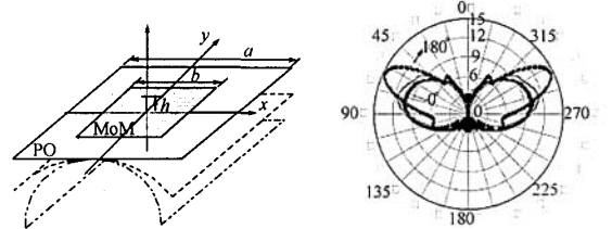
图 2 不同载体上的天线模型 图 3 不同载体上天线的特性比较 Fig.2 Antenna on different platform carrier Fig.3 Characters of antenna on different platform carrier
