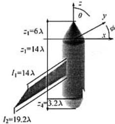
图 4 复杂载体上的天线模型 z Fig.4 Model of antenna on complicate platform
