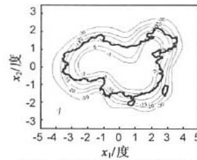
图 2 传统方法得到的赋形波束方向图
