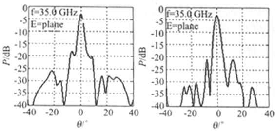
图2 辐射计天线 E 面、H 面功率方向图 Fig. 2 Antenna power pattern in E and H side for radiometer
