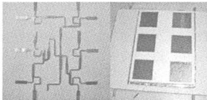
(a) 馈电功分网络 (b) 加工天线实物 图 6 天线加工实物
