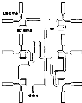
(b) 相移功分网图
