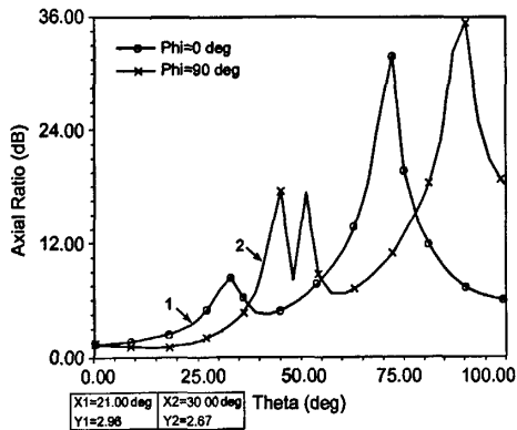
图5 天线在1590 MHz的广角轴比仿真结果
