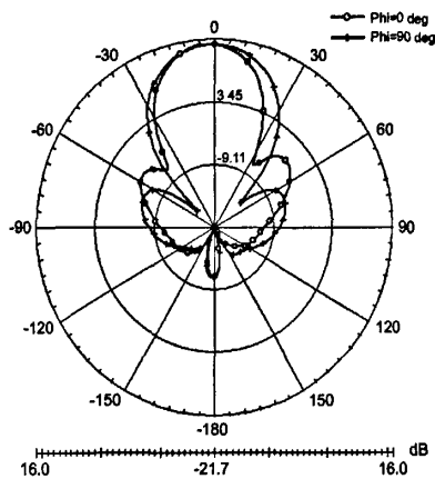
图4 天线在1590 MHz的增益方向性仿真结果
