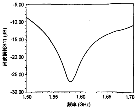
图3 天线回波损耗仿真结果
