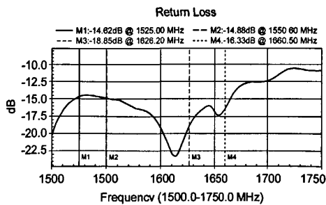
图 7 天线回波损耗测试结果
