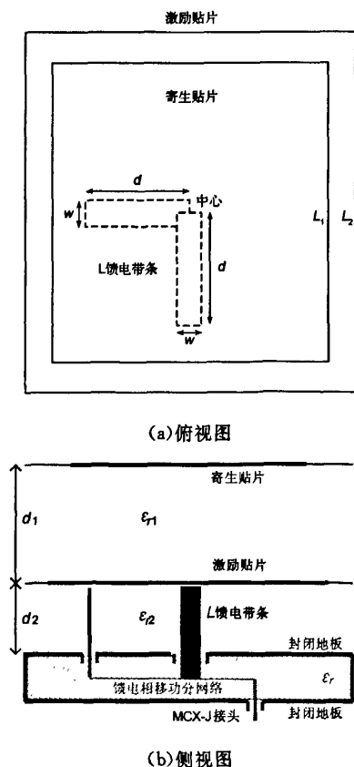
图1 单元天线结构示意图
