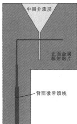
图1 渐变缝隙天线单元结构模型图
