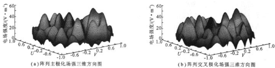
图 5 阵列场强三维方向图
