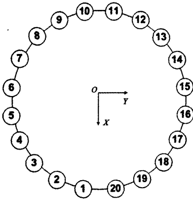
图 3 20 单元介质锥台共性阵列单元排布示意图
