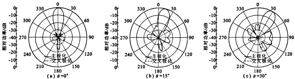
图 7 PSO 优化波束扫描至不同角度时的归一化方向图
