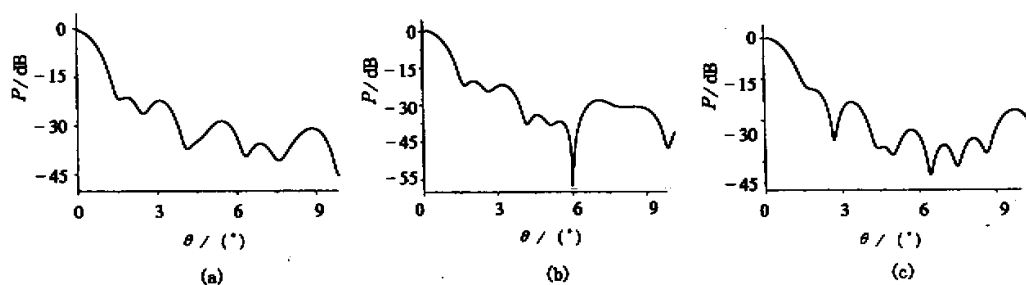
图5 加入馈源后天线的远场方向图
