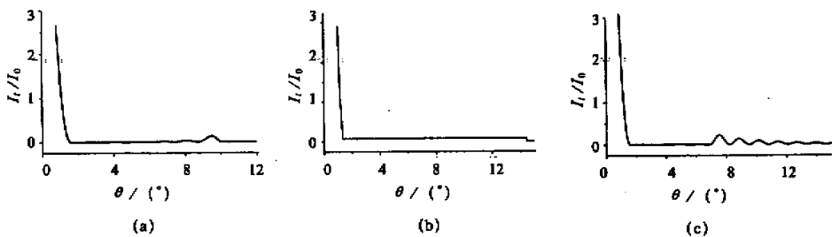
图 2 根据降低第一旁瓣电平要求所采用的 3 种目标衍射分布 (a) 逆旁瓣分布 (b) 平坦分布 (c) 近旁瓣抑制远旁瓣提升分布
