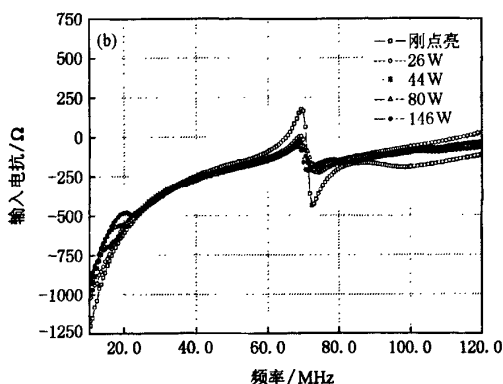
图4 不同激励功率条件下等离子体天线输入阻抗 (a)实部; (b)虚部
