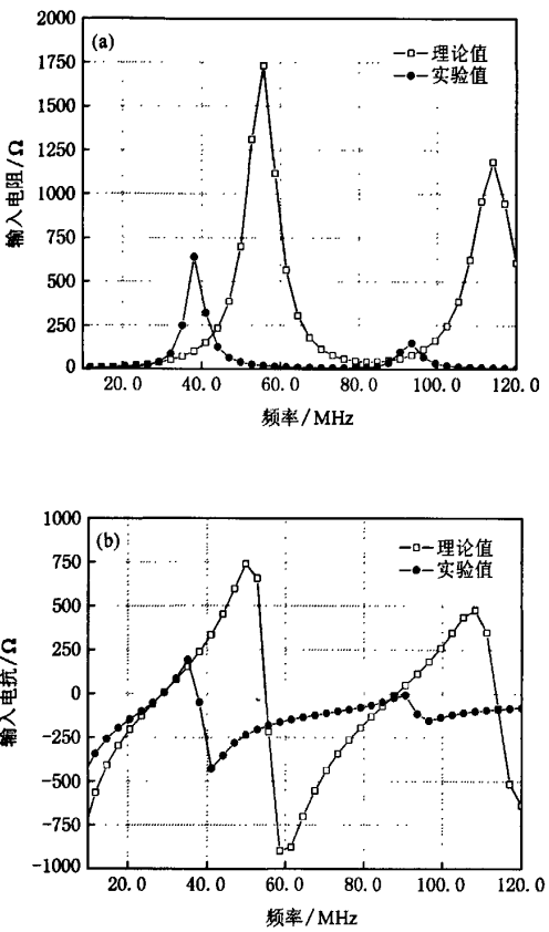
图 5 腔体中铜管与单极天线理论输入阻抗比较 (a)实部;(b)虚部
