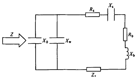
图3 柱形等离子体天线系统等效电路
