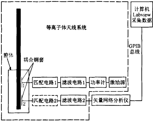
图 2 等离子体天线系统输入阻抗测量原理框图
