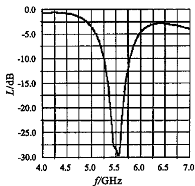
(a) 反射系数与频率的关系图
