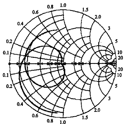
(b) 导纳圆图
