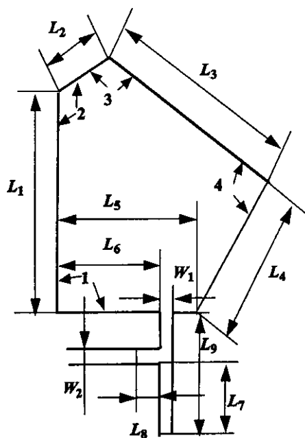
图 3 天线各边及馈线尺寸
