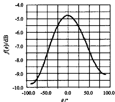
(c) \theta 方向图
