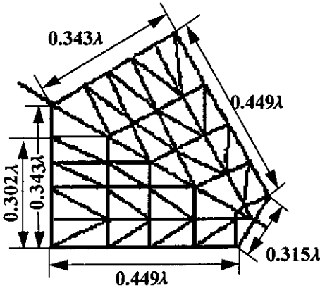
图 2 五边形微带天线的单元划分
