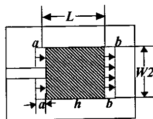
图 1 矩形微带天线的场图
