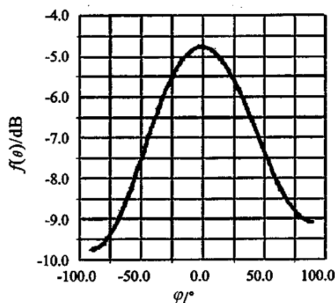
(d) 方向图
