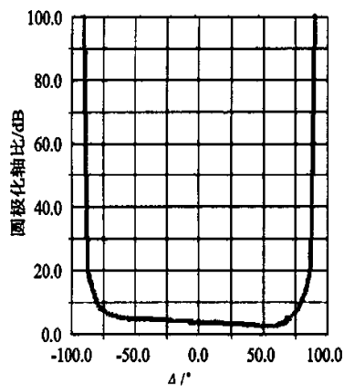
(e) 轴比图
