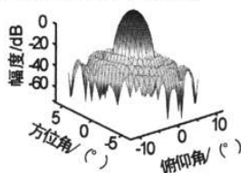
图4 天线的三维方向图
