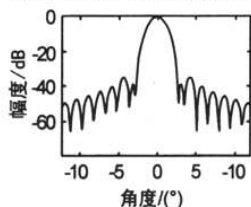
图3 天线的二维方向图
