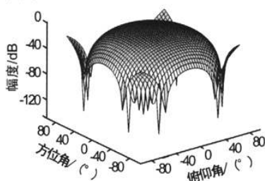
图2 馈源辐射初级方向图
