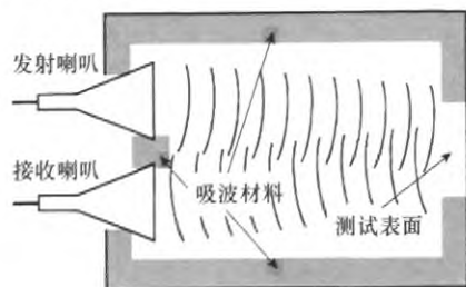
图 9 RCS 缩减测试示意图
