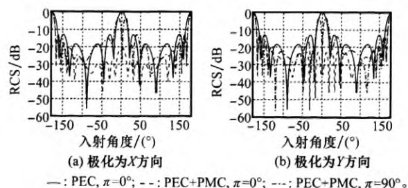
图 5 金属和 PEC+PMC 组合结构在不同极化下的 RCS
