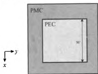
图 7 环形结构的 PMC 与 PEC 组合表面
