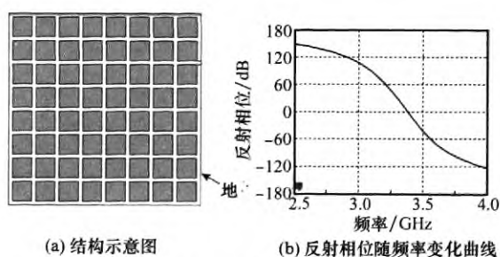
图 1 周期排列的 AMC 结构示意图以及反射相位随频率变化曲线
