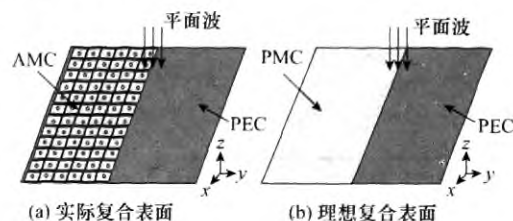
图 3 AMC+PEC 的复合表面
