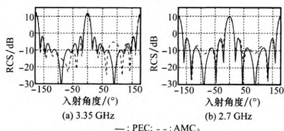
图 2 AMC 结构与相同尺寸金属板的 RCS 对比
