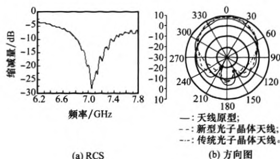
图 11 天线 RCS 和方向图测试结果
