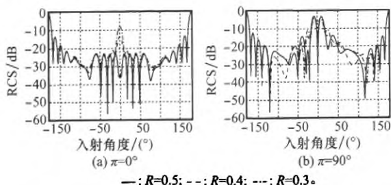
图 6 金属和 PEC+PMC 组合结构在不同 R 值下的 RCS
