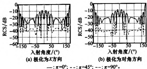
图 8 环形结构的复合表面 RCS
