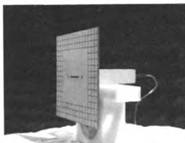
图 10 加载复合表面的波导缝隙天线
