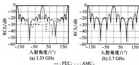
图 4 X 极化入射波在 \pi=0 面的复合表面与金属面 RCS 计算结果
