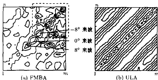
图 3 不相关来波时, 两种阵列输出协方差矩阵元素的幅度
