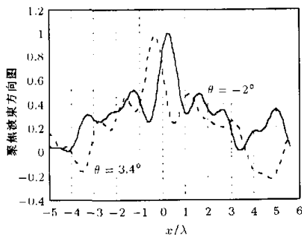
图2 FZP 聚焦平面上的一组聚焦场分布
