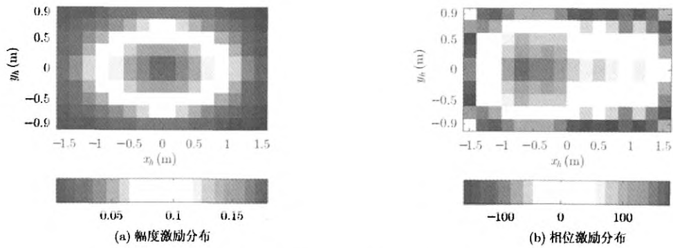
图 4 E 面余割平方波束的激励分布
