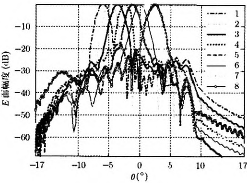
图 5 扫描波束的 E 面方向图
