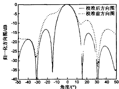
图1 校准前后的天线方向图
