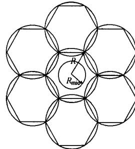
图2 嵌入波束结构
