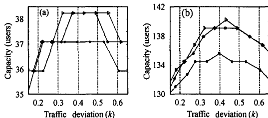
图7(a) G_p=128 (IS-95)系统容量随 k 变化图 (b) G_p=480 (UMTS)系统容量随 k 变化图 Fig.7 (a) G_p=128 (IS-95) Capacity vs. k (b) G_p=480 (UMTS) Capacity vs. k
