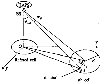
图3 HAPS 区间干扰几何关系
