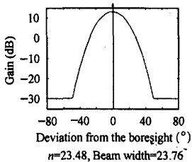
图1 天线方向图
