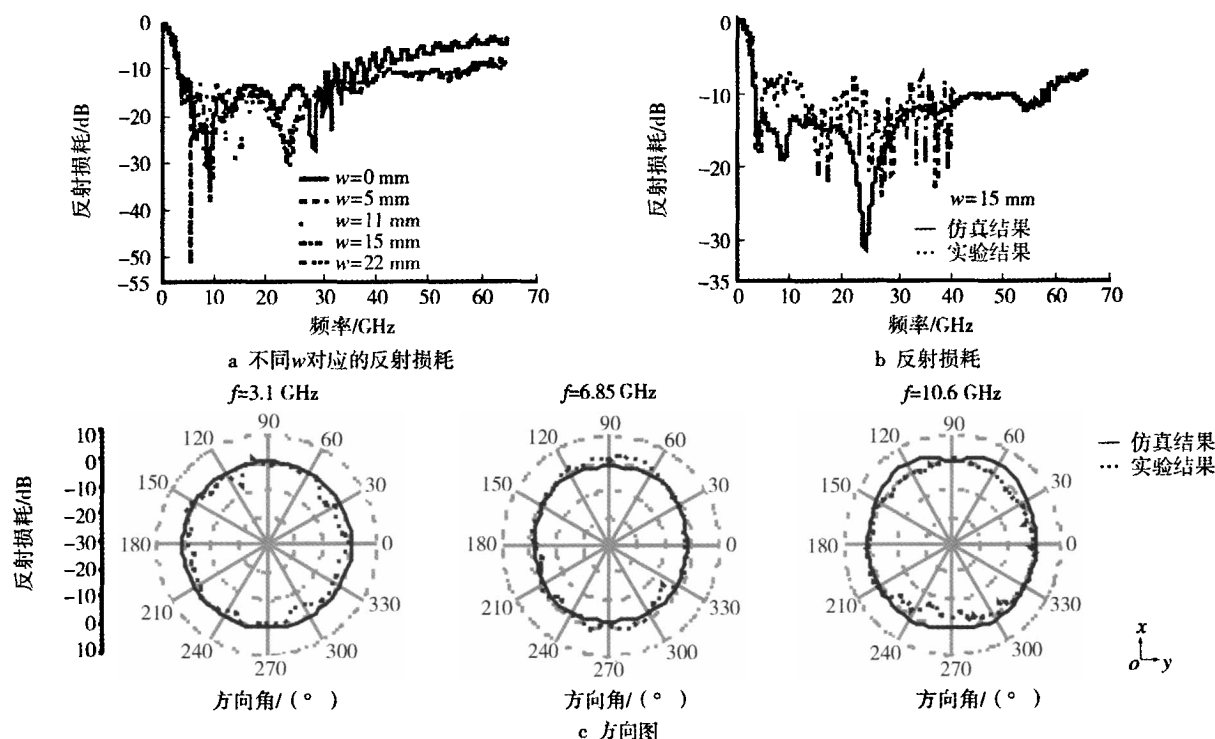
图6 折叠圆片单极天线的性能
