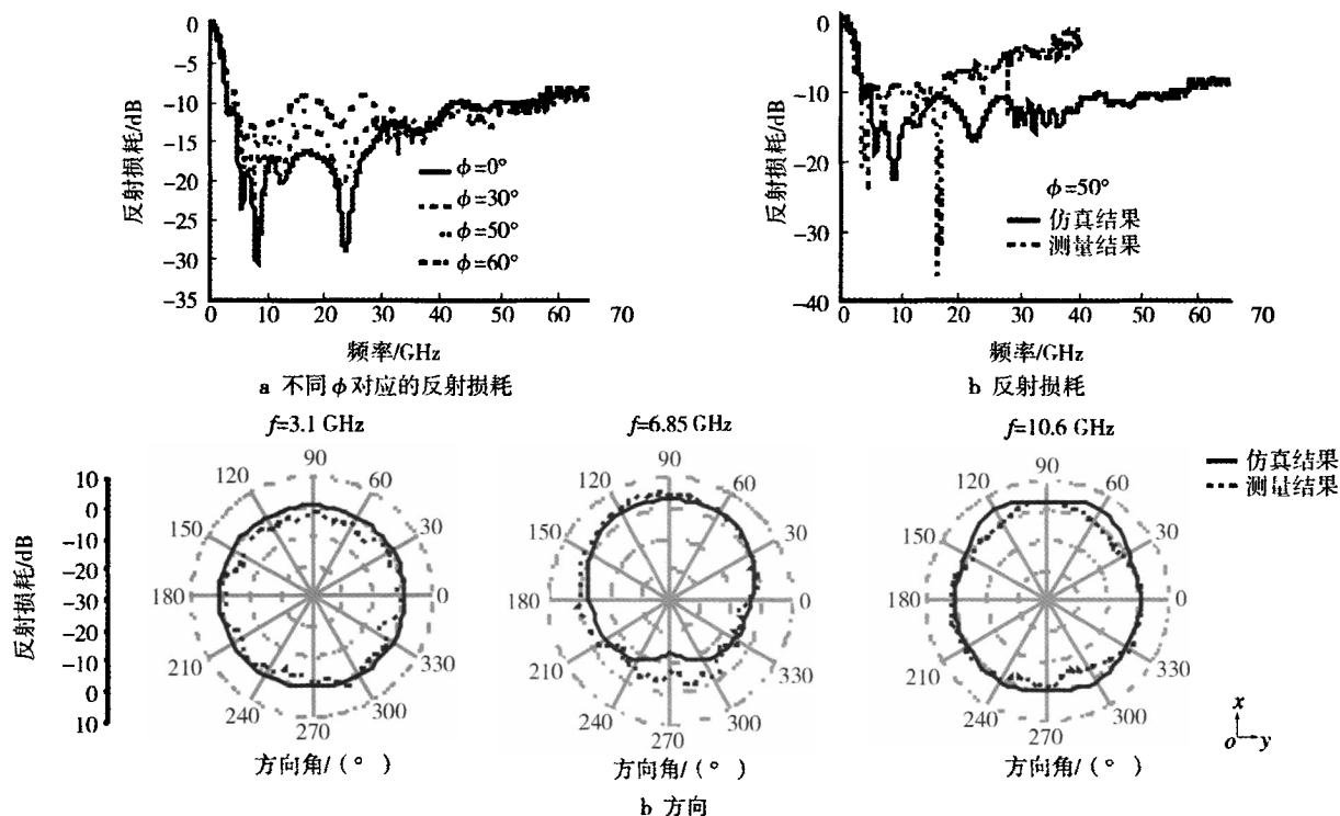
图8 弯角结构圆片单极天线的性能
