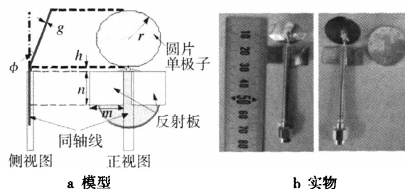
图7 弯角结构的圆片单极天线
