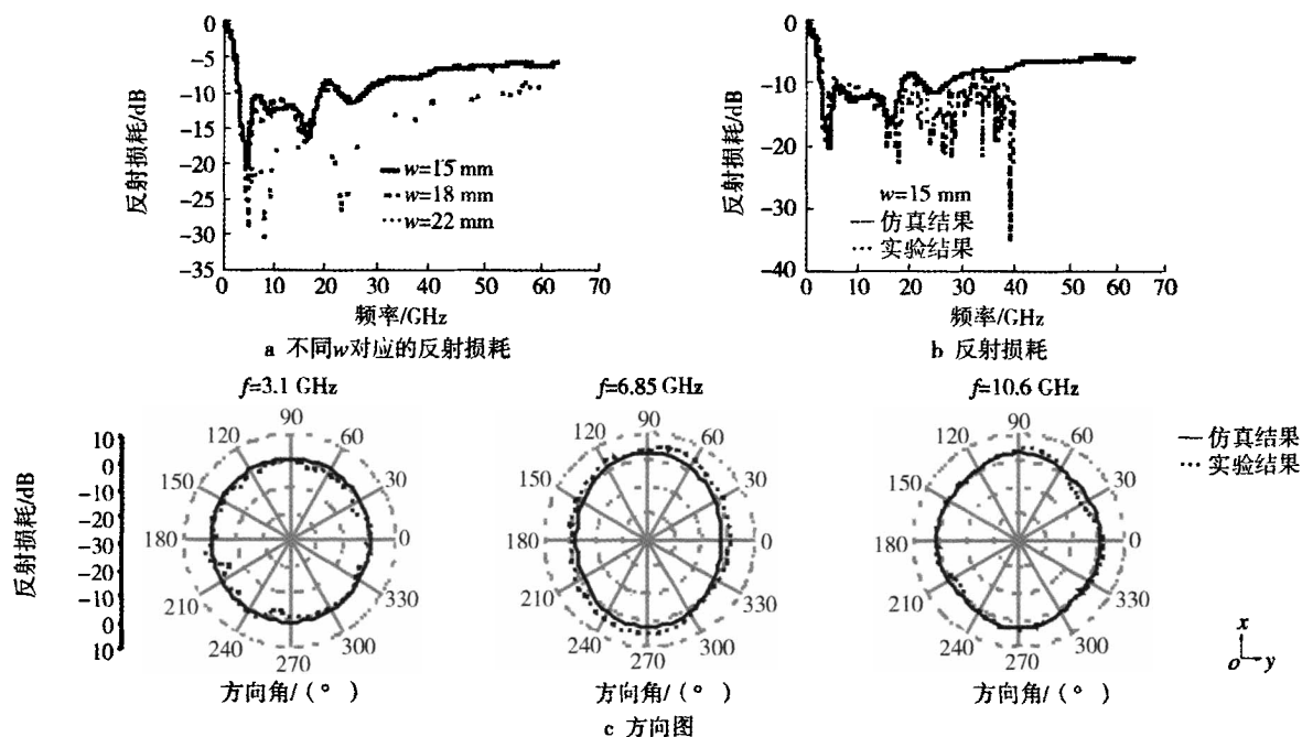
图4 剪切平板圆片单极天线的性能
