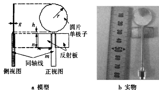
图1 平板圆片单极天线
