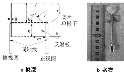
图3 剪切平板圆片单极天线
