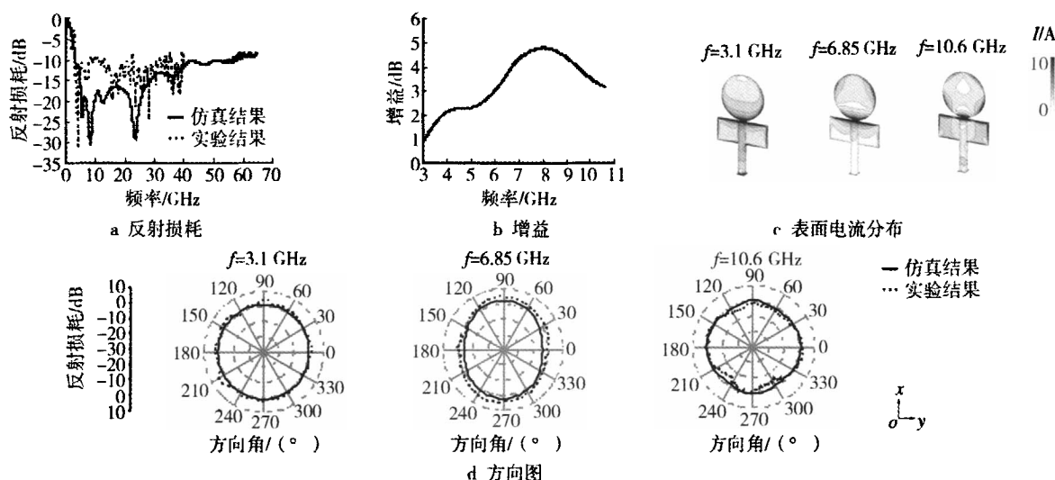
图2 平板圆片单极天线的性能
