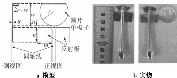
图5 折叠圆片单极天线
