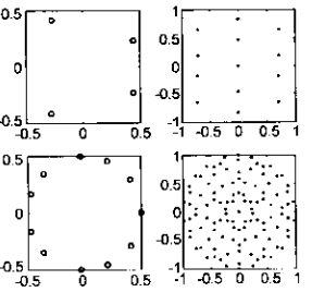
图5 全圆周天线单元结构分布及其频谱图
