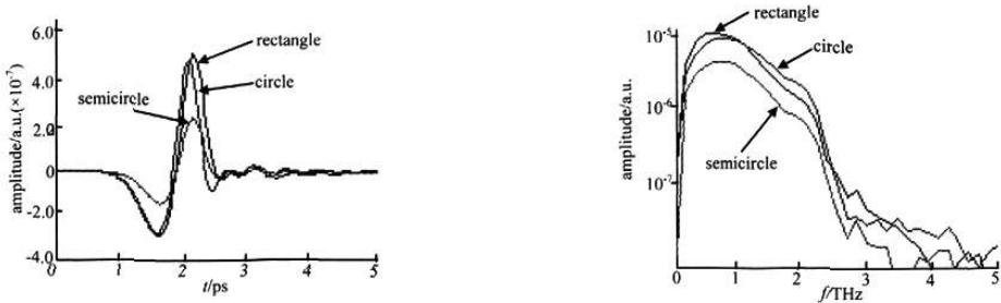
Fig.5 THz time domain waveform and frequency of PCAs with different electrode shapes 图 5 不同形状的光导天线产生的 THz 波的时域波形和频谱
