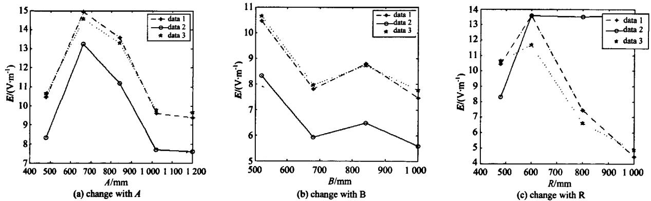
Fig.9 Variety of the far-field radiation 图 9 主轴远场辐射值的变化
