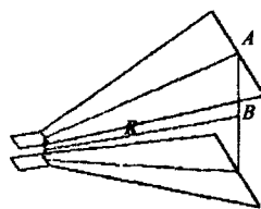
Fig.2 Structure of TEM horn 图 2 TEM 喇叭模型图
