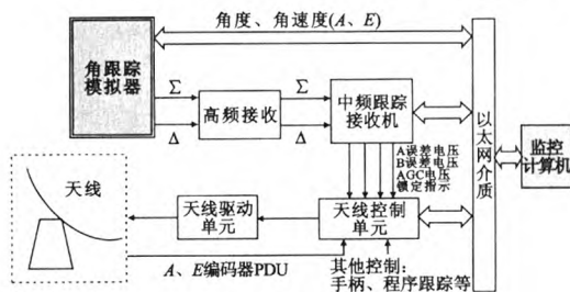
图 1 角跟踪模拟器工作原理框图
