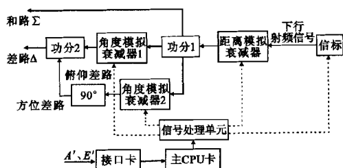
图4 角误差信号模拟原理框图
