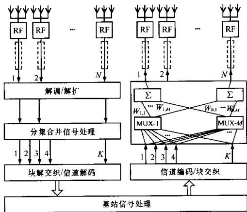
图1 CCSDA 结构示意图
