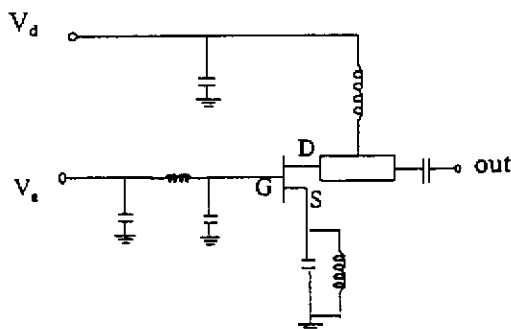
图3 单片 18GHz 振荡器等效电路图
