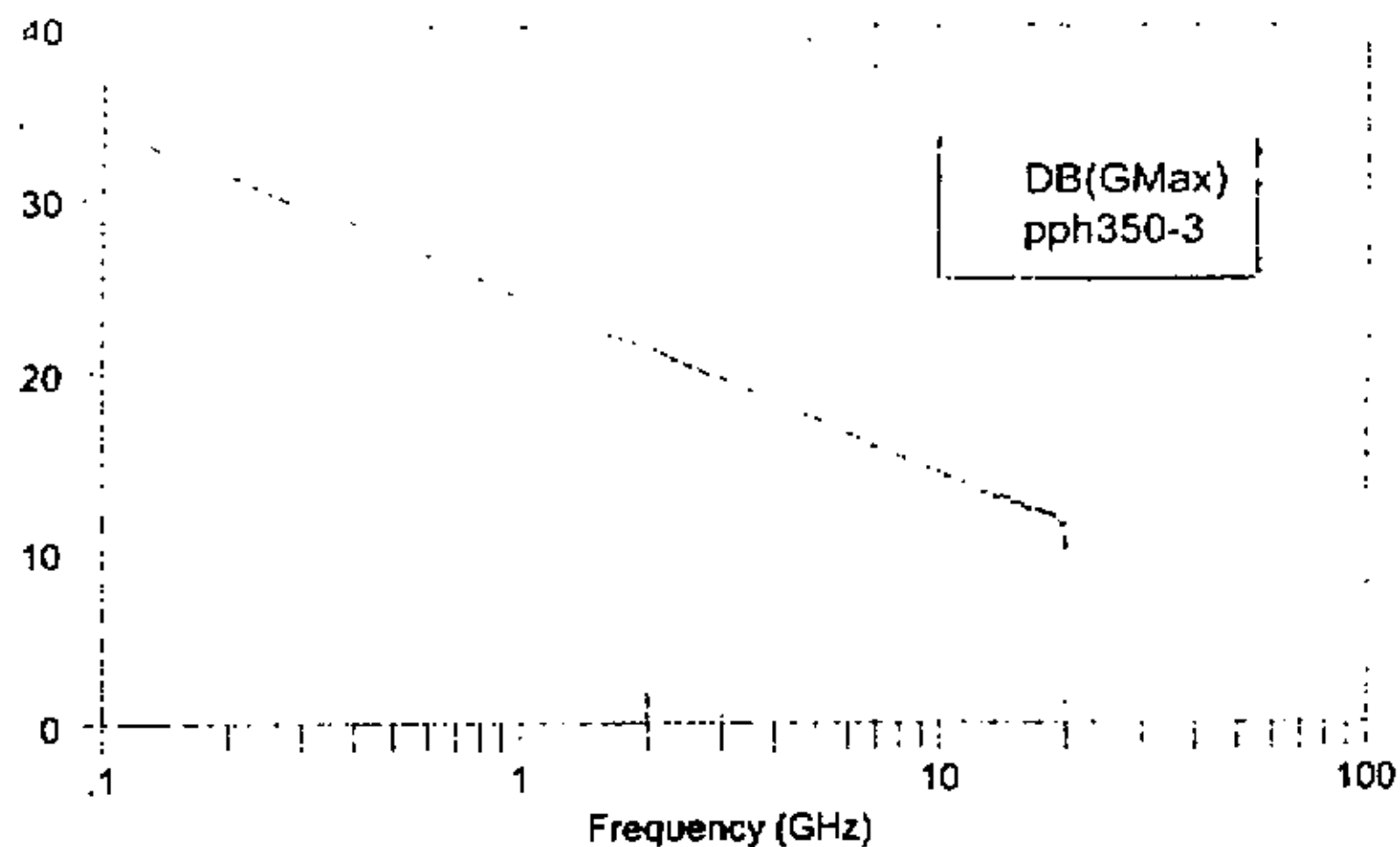
图2 PHEMT 最大可用增益推算结果
