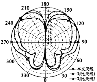
图 9 天线 E 面归一化辐射方向图(2 170 MHz) Fig. 9 The normalized radiation pattern in E-plane(2 170 MHz)
