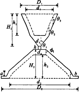
图3 优化天线结构示意图 Fig. 3 The structural diagram of optimized antenna
