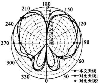
图 11 天线 E 面归一化辐射方向图(2 500 MHz) Fig. 11 The normalized radiation pattern in E-plane(2 500 MHz)
