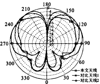
图 10 天线 E 面归一化辐射方向图(2 300 MHz) Fig. 10 The normalized radiation pattern in E-plane(2 300 MHz)
