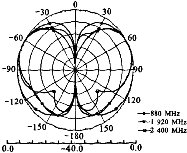
图4 天线E面归一化辐射方向仿真图 Fig. 4 The normalized radiation pattern in E-plane
