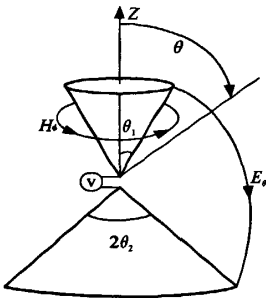
图2 不对称双锥天线 Fig. 2 Asymmetrical biconical antenna
