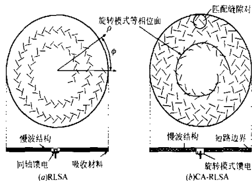
图1 RLSA和CA-RLSA结构示意图
