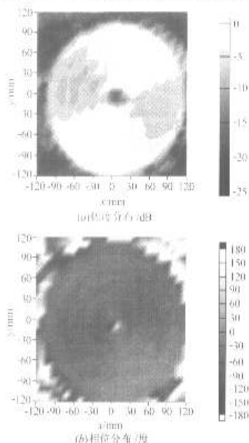
图 4 CA-RLSA 口面场分布测量值
