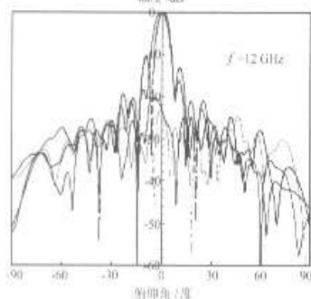
图 5 CA-RLSA 辐射方向图测量结果
