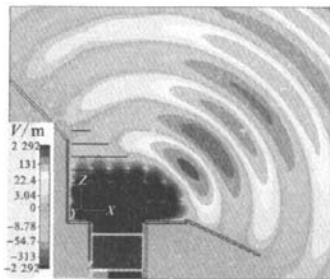
图6 劈尖波导实验
