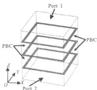
图3 结构单元仿真模型
