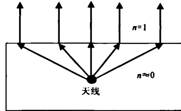
图2 嵌入零折射率超材料偶极子天线
