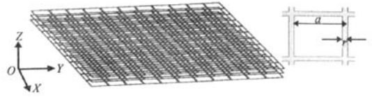
图1 零折射率超材料结构图
