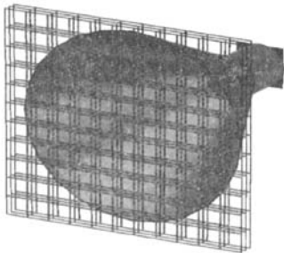
图 10 加载零折射率超材料喇叭天线模型 Fig. 10 Model of the horn antenna with ZIM
