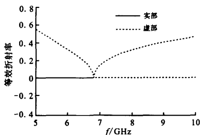
图5 等效折射率
