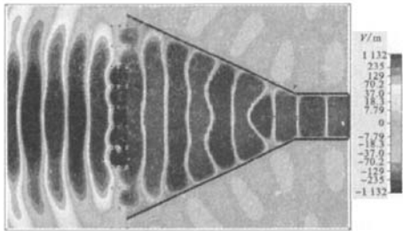
图 11 加载零折射率超材料后喇叭天线在 7.1 GHz 的电磁分布图 Fig. 11 Electric field distribution of the horn antenna with ZIM at 7.1 GHz
