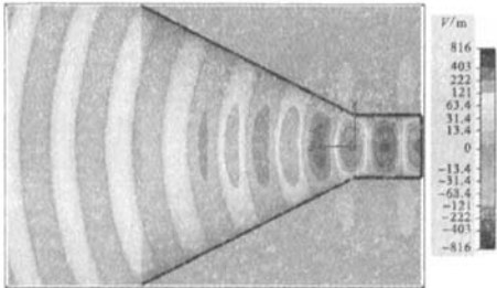
图 8 喇叭天线在 7.1 GHz 的电场分布 Fig. 8 Electric field distribution of the horn antenna at 7.1 GHz
