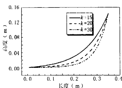
图5 天线指数渐变曲边
