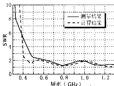
图4 天线工作频带内的驻波比
