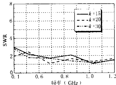
图6 不同变化率对应的天线驻波
