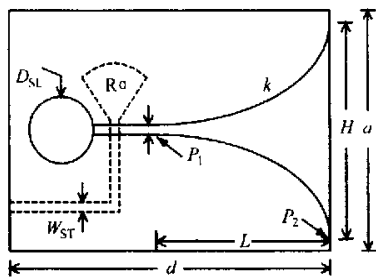
图 1 指数渐变开槽天线结构
