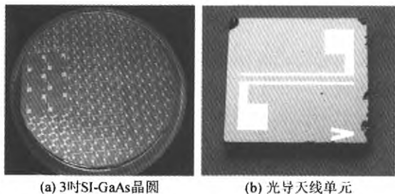
图1 SI-GaAs 光导天线
