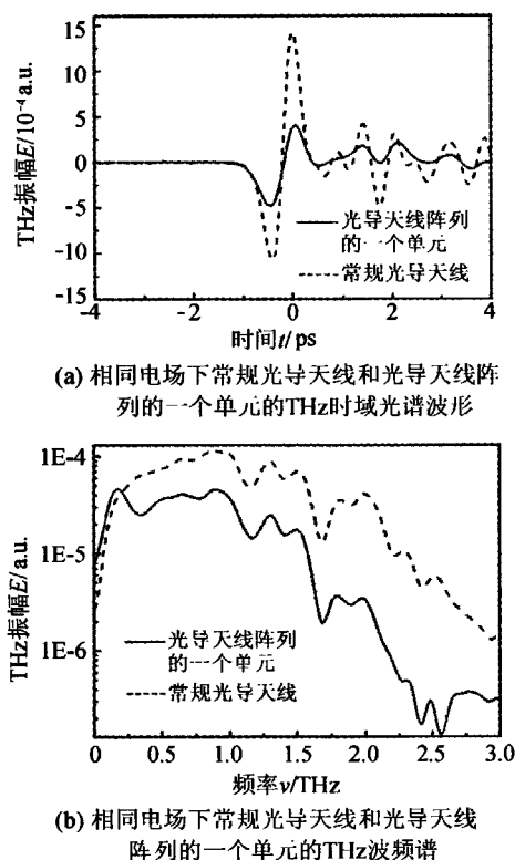
图5 常规光导天线与光导天线阵列的一个单元的 THz 辐射
