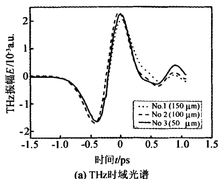
图 3 天线 No. 1、No. 2、No. 3 的 THz 时域光谱及傅里叶变换频谱
