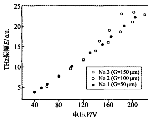
图 4 THz 振幅与天线 No. 1、No. 2 以及 No. 3 外加偏置电压之间的关系
