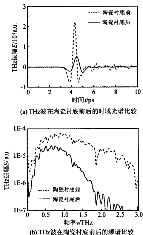
图6 THz 波在陶瓷衬底前后的比较
