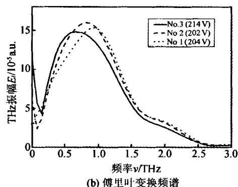
图 3 天线 No. 1、No. 2、No. 3 的 THz 时域光谱及傅里叶变换频谱
