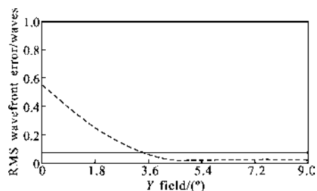
图 11 离轴三反系统的均方根波前误差图
