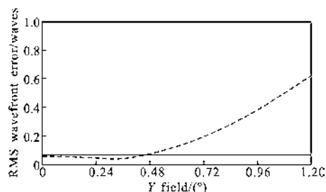
图 10 卡式同轴两反系统的均方根波前误差图
