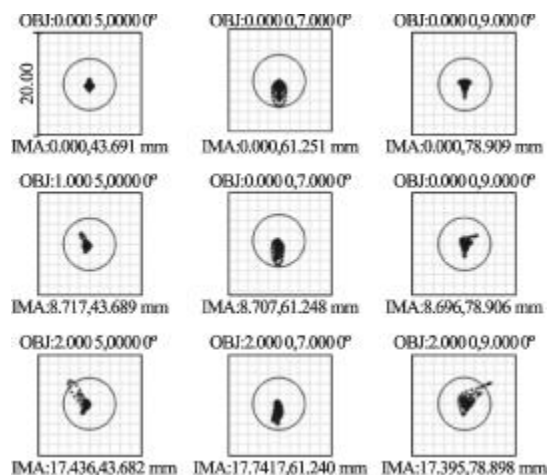
图7 离轴三反系统的点列图
