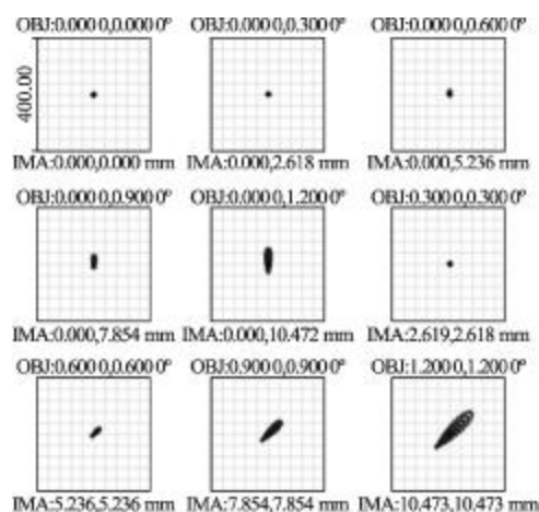
图6 卡式同轴两反系统的点列图
