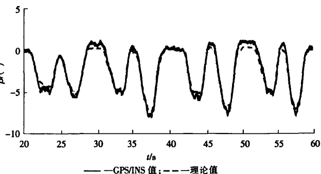
图 3 转向时的车辆侧偏角测量值和理论值
