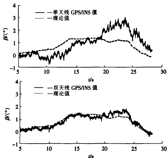
图 4 GPS/INS 系统估计的车辆侧偏角
