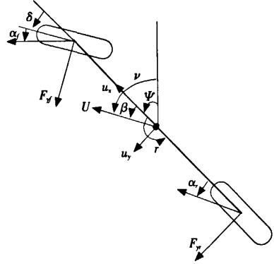
图 1 汽车二自由度动力学模型示意图
