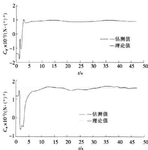
图7 双天线 GPS/INS 系统估测的轮胎侧偏刚度
