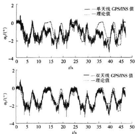
图5 GPS/INS系统估测的前轮侧偏角
