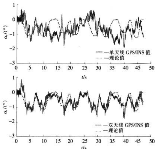
图6 GPS/INS系统估测的后轮侧偏角
