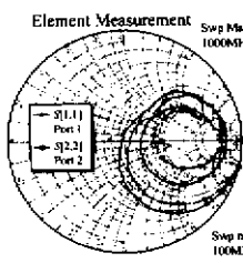
图4 多偶极子小天线端口阻抗特性
