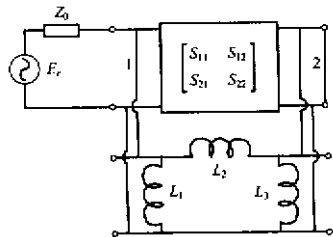
图3 多偶极子小天线阻抗匹配电路原理图. L_1 = 60\text{nH} , L_2 = 108\text{nH} .
