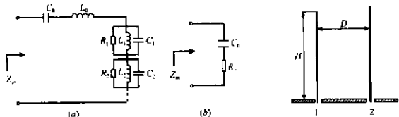
图1 (a) 偶极子天线的等效电路 (b) 电小天线在低频端的等效电路
