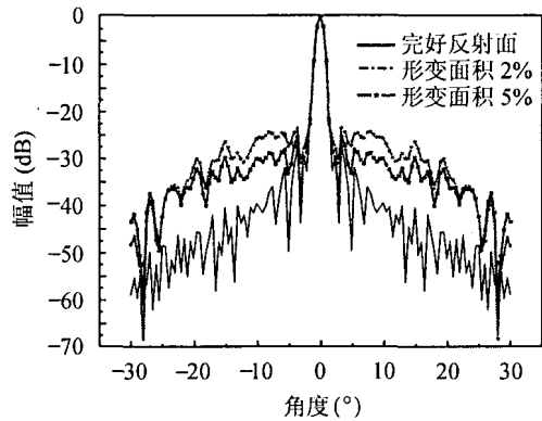
图 4 水平面方向图
