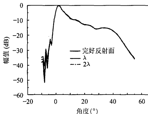
图 5 垂直面方向图
