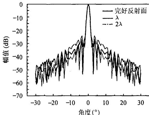
图 6 水平面方向图
