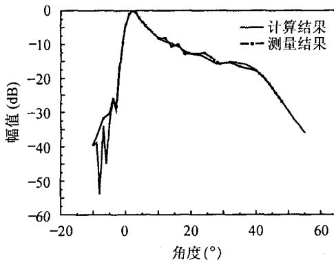
图 1 垂直面方向图
