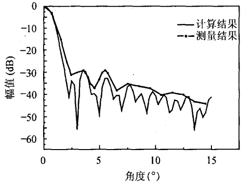
图 2 水平面方向图
