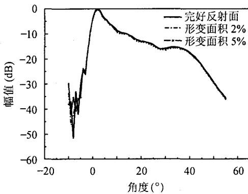
图 3 垂直面方向图
