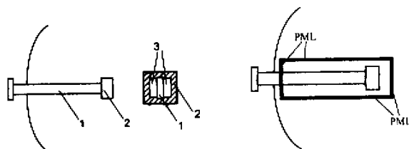
图1 波导缝隙馈电抛物面天线 (1) 馈电波导 (2) 背腔 (3) 辐射缝对
