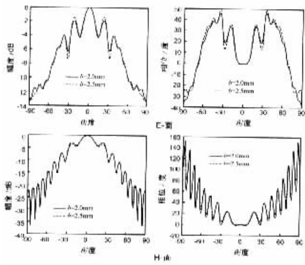
图 5 馈源辐射缝为圆弧缝时的馈源幅相方向图。
