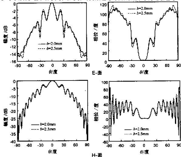
图 4 馈源辐射缝为直缝时的馈源幅相方向图.
