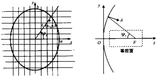
图 3 抛物面上电流计算坐标
