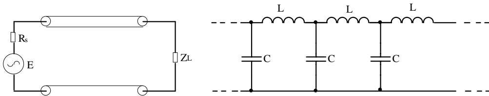
传输线的等效电路
