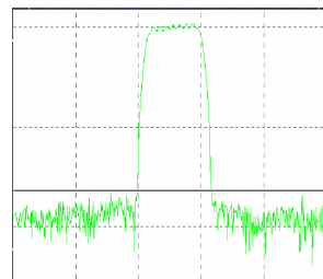
幅频特性
