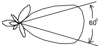
水平方向图
