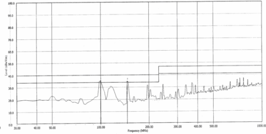
天线垂直极化方向
