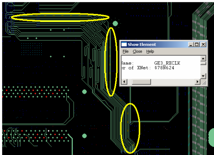
图 10 单板布线
