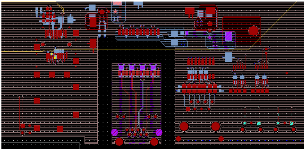
图 5 单板布线
