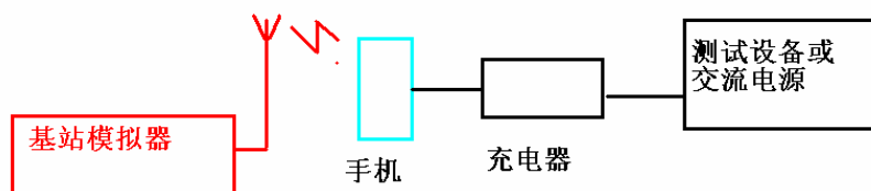
图 1 手机测试连接方式
