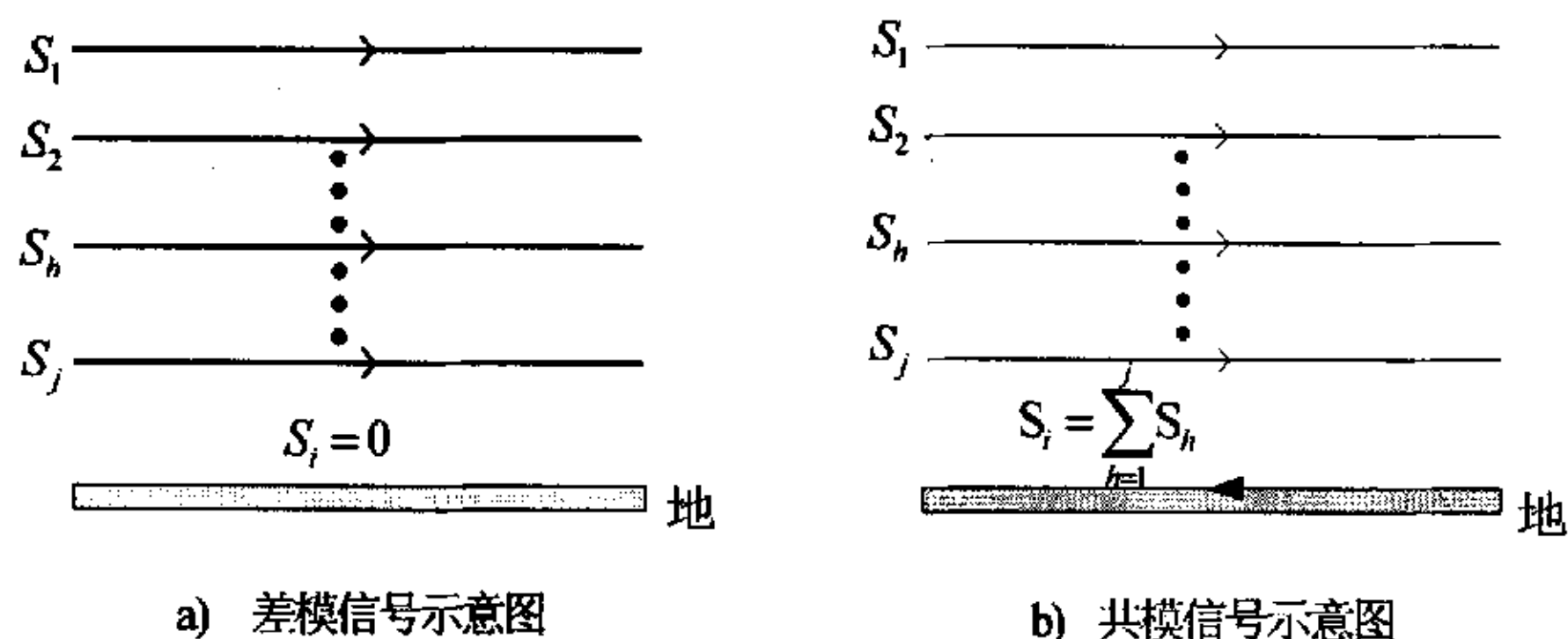
图 2-4 共模和差模信号流经路线
